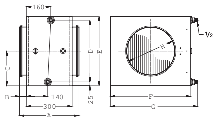
Нагреватель \varnothing 400 мм для CDP 75 и 125
