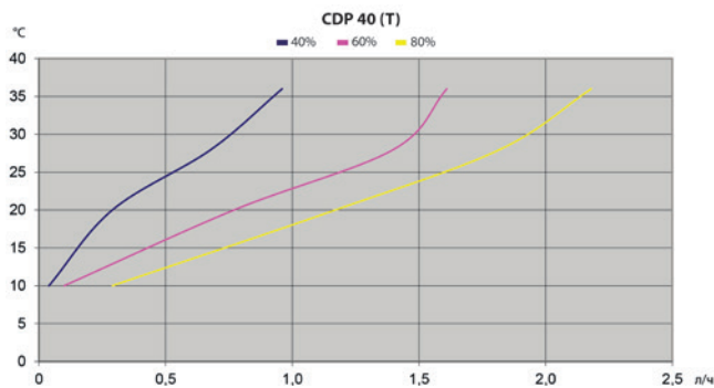
Удельное энергопотребление 0,47 кВт*ч/л при 28°C / 60% отн.влажности
