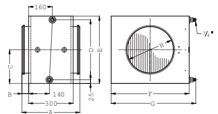
Нагреватель \varnothing 500 мм для CDP 165
