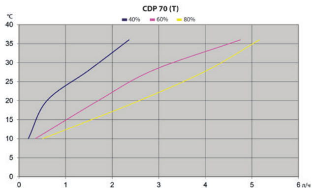
Удельное энергопотребление 0,43 кВт*ч/л при 28°C / 60% отн.влажности
