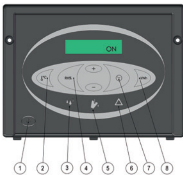
Панель управления
