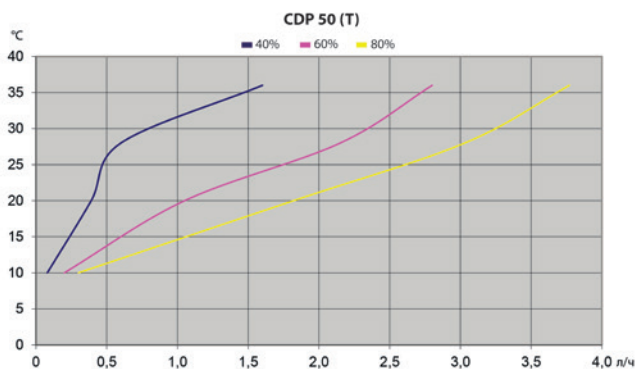
Удельное энергопотребление 0,48 кВт*ч/л при 28°C / 60% отн.влажности
